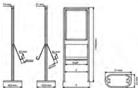
Doppelseitige Prospektablage für 3 x DIN A4.
